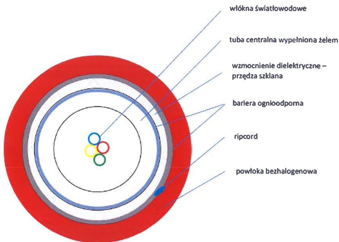
Rys. nr 1 Przekrój osiowy kabla światłowodowego typu BITfiber Flame CLT
